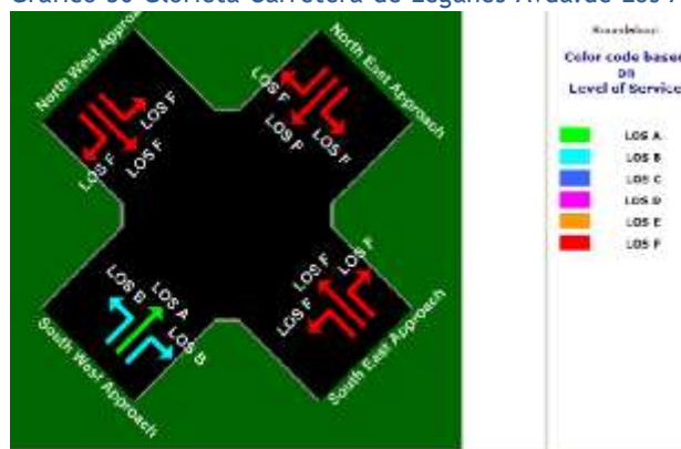
Gráfico 30 Glorieta Carretera de Leganés-Avda.de Los Andes. Periodo Punta Mañana.
